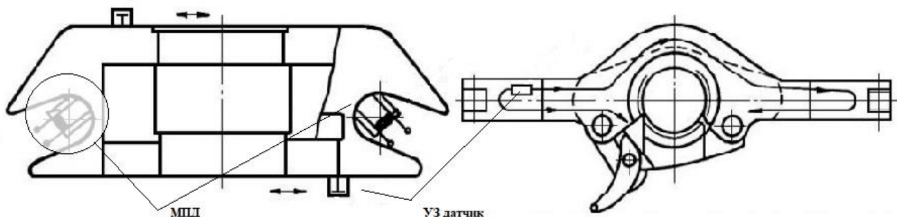
Схема контроля:
